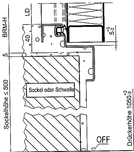
Ausführungsvariante: Zarge 4-seitig umlaufend
