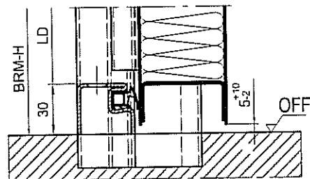
Ausführungsvariante: Schwelle mit Auflaufprofil
