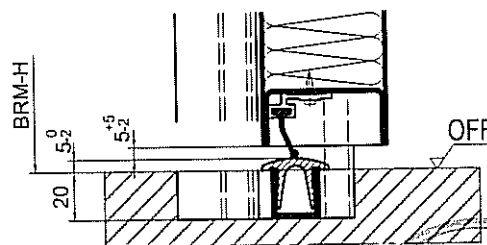
Ausführungsvariante: Schwelle mit Auflaufprofil
